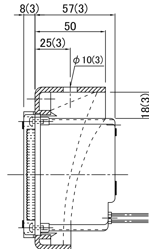
“A-A”断面
