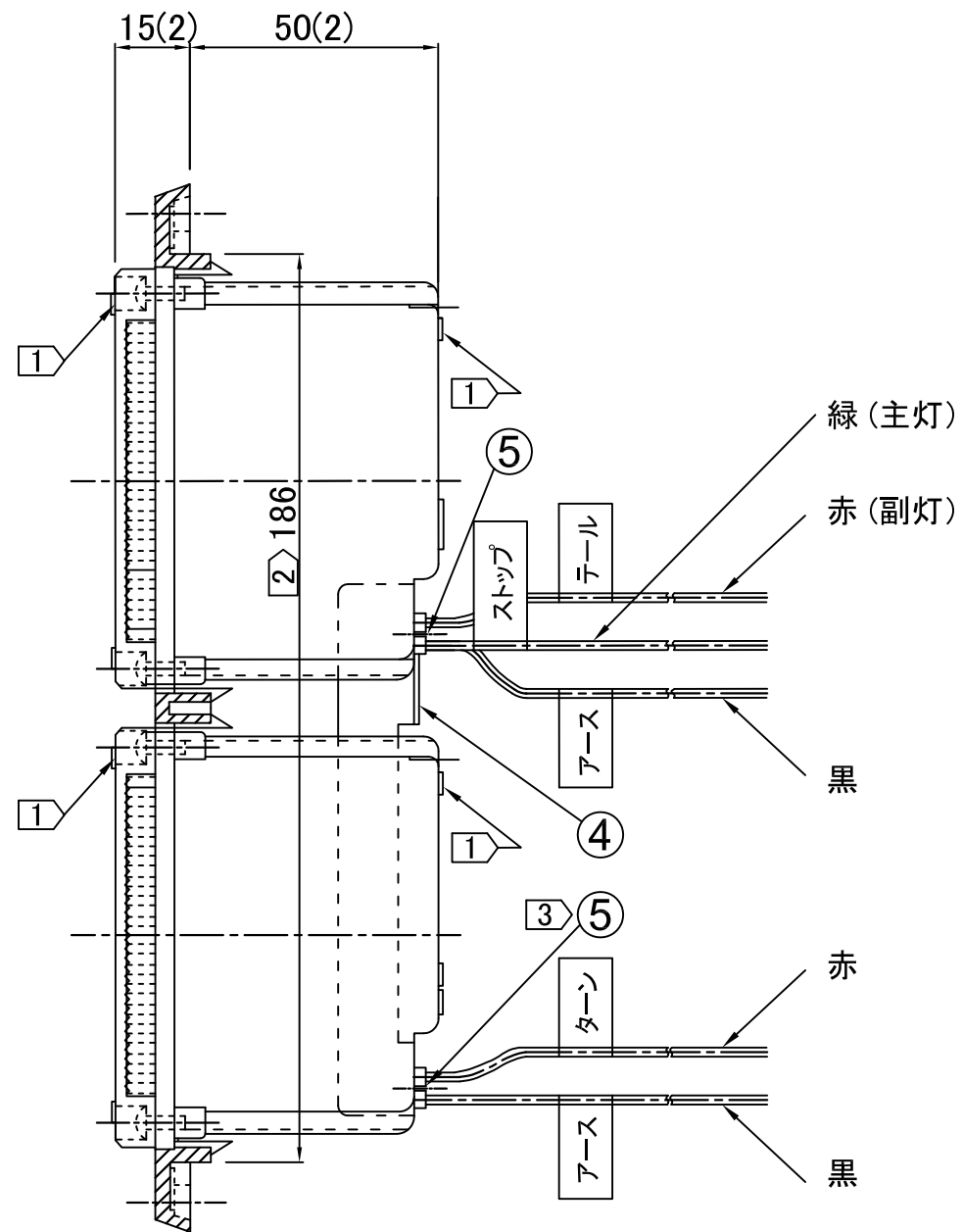
"A-A" 断面
