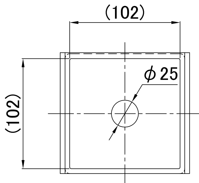
A 矢視図
