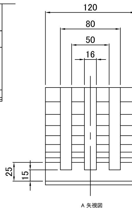
A 矢视图
