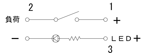
回路図
