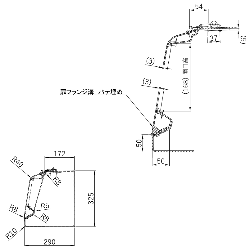
A-A断面図(FREE)
