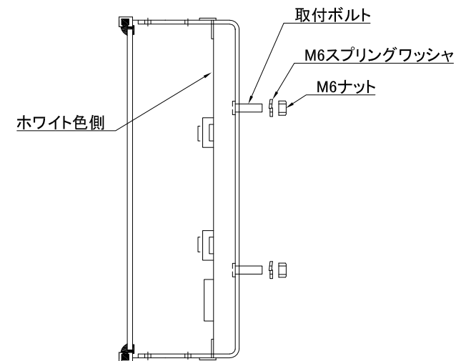
断面拡大図
