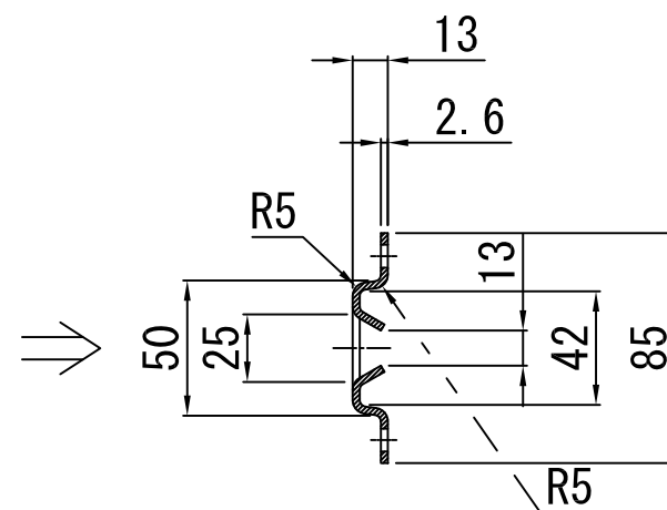
B-B矢視図
