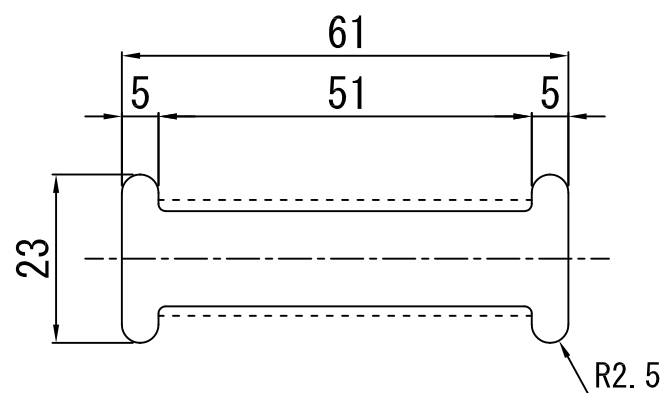
切り込み加工部詳細 (S=1/1)
