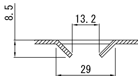
A-A矢视图(S=1/1)
