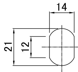
A-A 断面图
