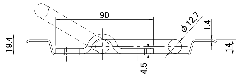
A-A 断面図
