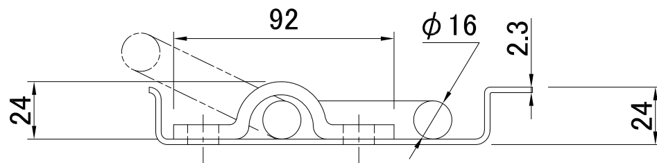
A-A 断面图
