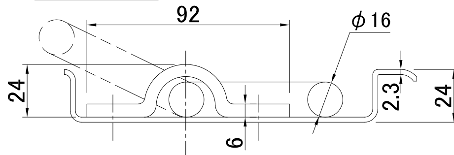
A-A 断面图
