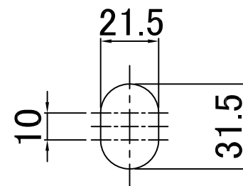
長孔詳細図
