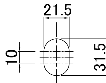
長孔詳細図
