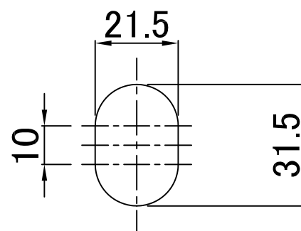
長孔詳細図
