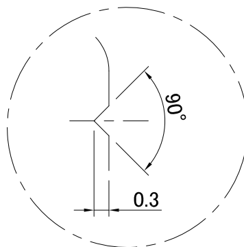
A部詳細(10:1)
