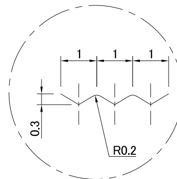
B部ローレット詳細(10:1)
