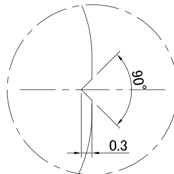
A 詳細 (10:1)
