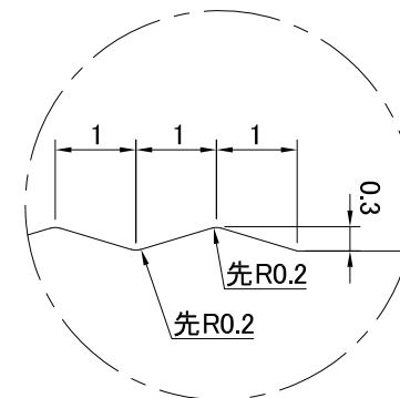
B ローレット部詳細 (10:1)
