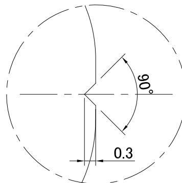
A 詳細(10:1)
