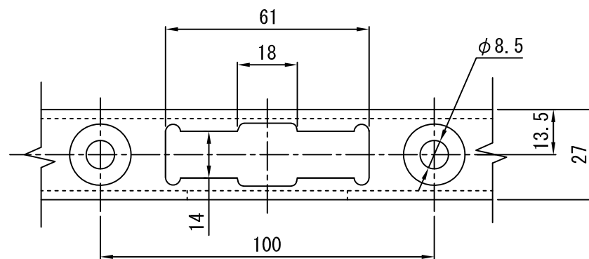
溶接部詳細図 (S=1/1)
