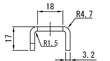
B-B断面詳細図 (S=1/1)
