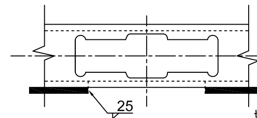
溶接部詳細図 (S=1/1)
