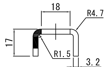
B-B断面詳細図 拡大
