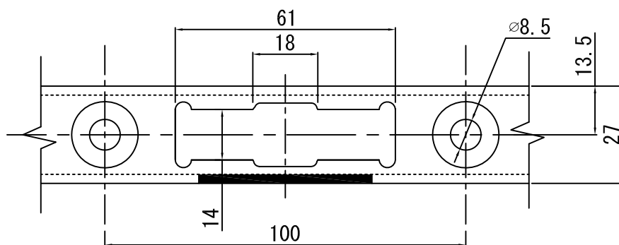
A部詳細図拡大
