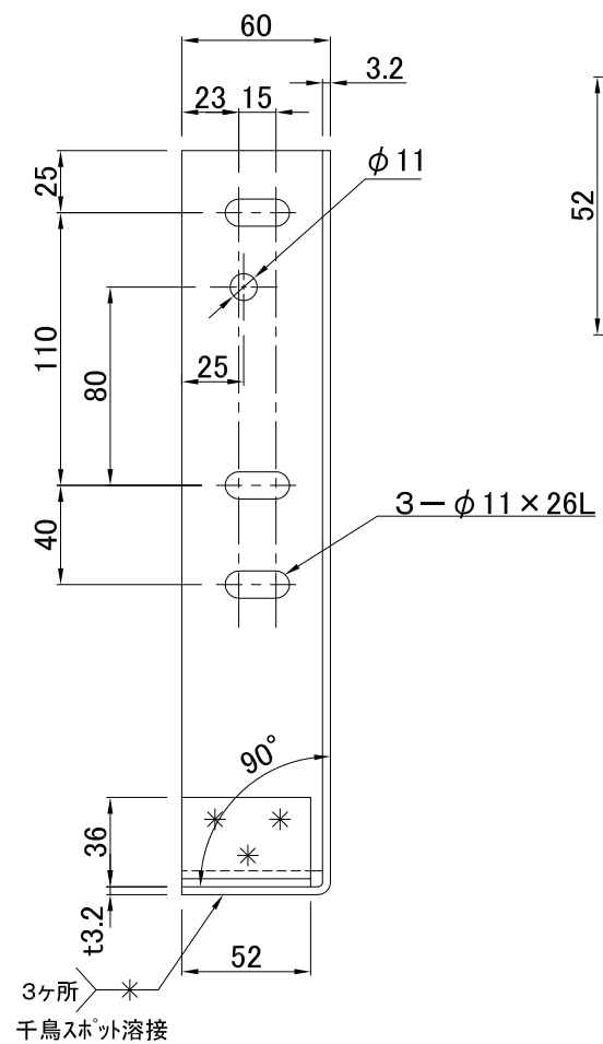
2. 補強詳細図 (拡大図)
