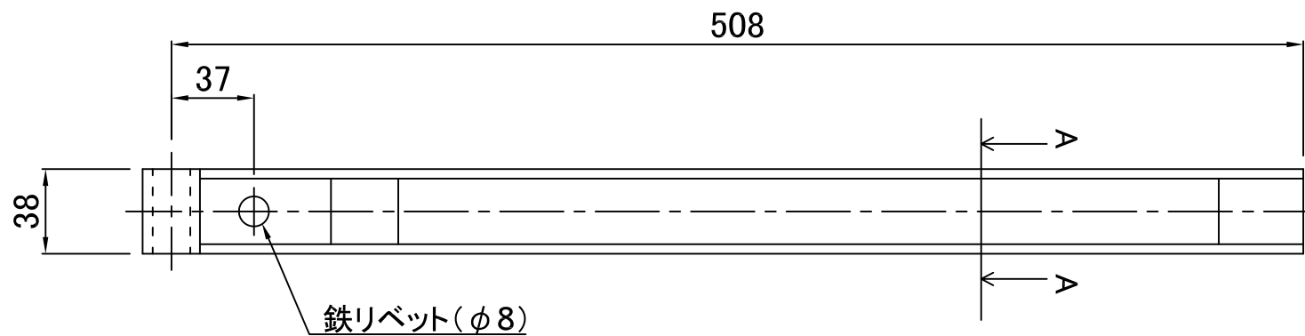
鉄リベット図 (FREE)
