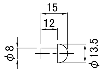
鉄リベット図 (FREE)
