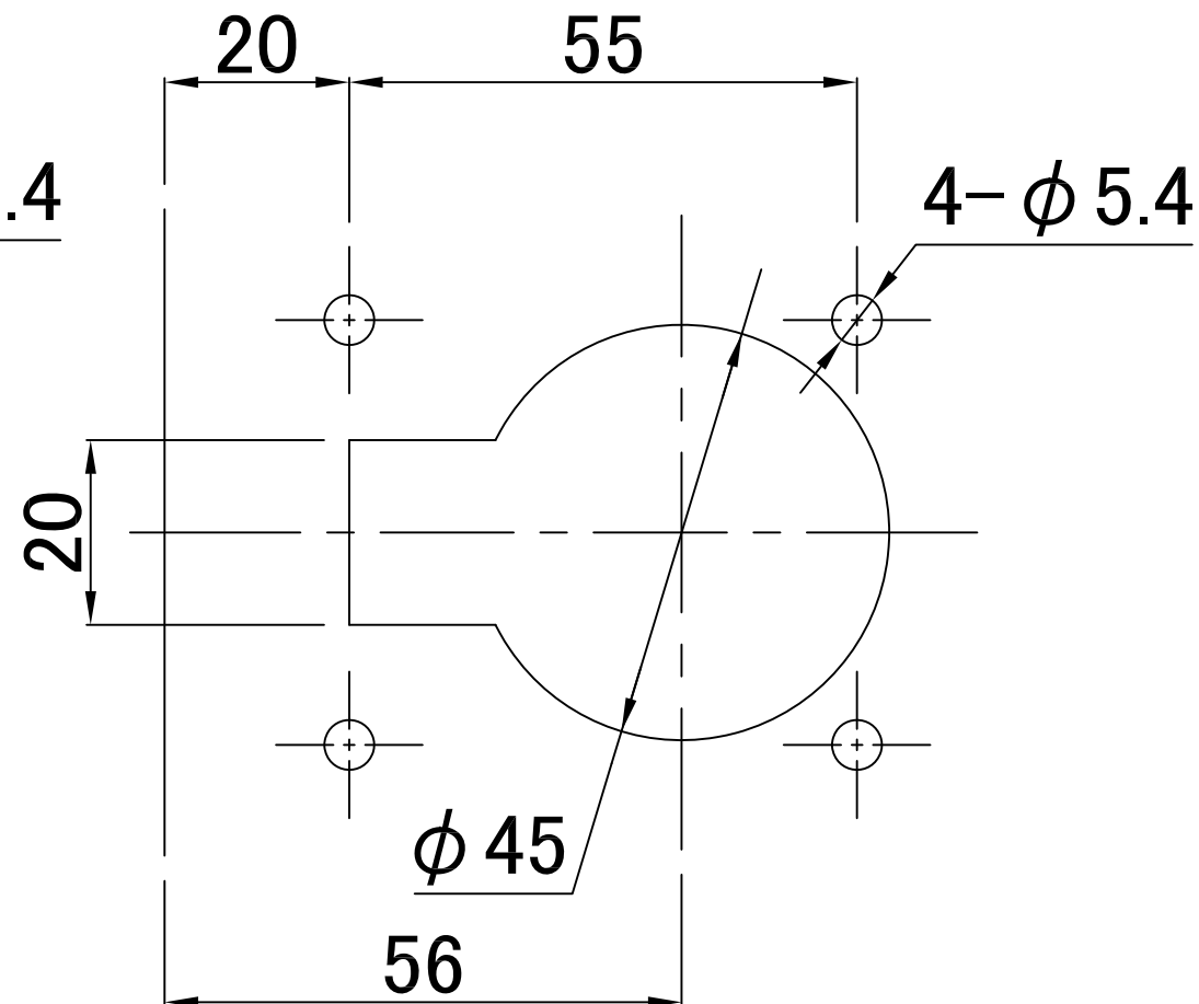
裏面から取付ける場合
