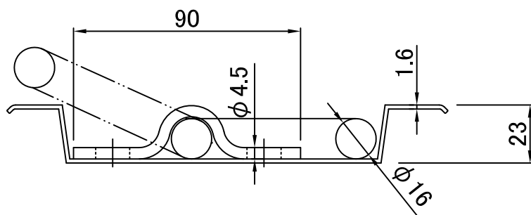
A-A 断面図
